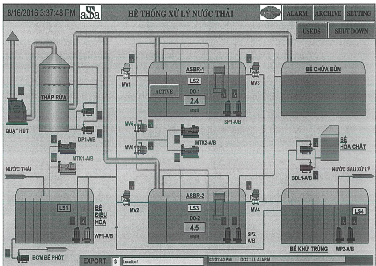
Hình 3. Hệ thống theo dõi tự động quá trình xử lý nước thải tại bệnh viện
