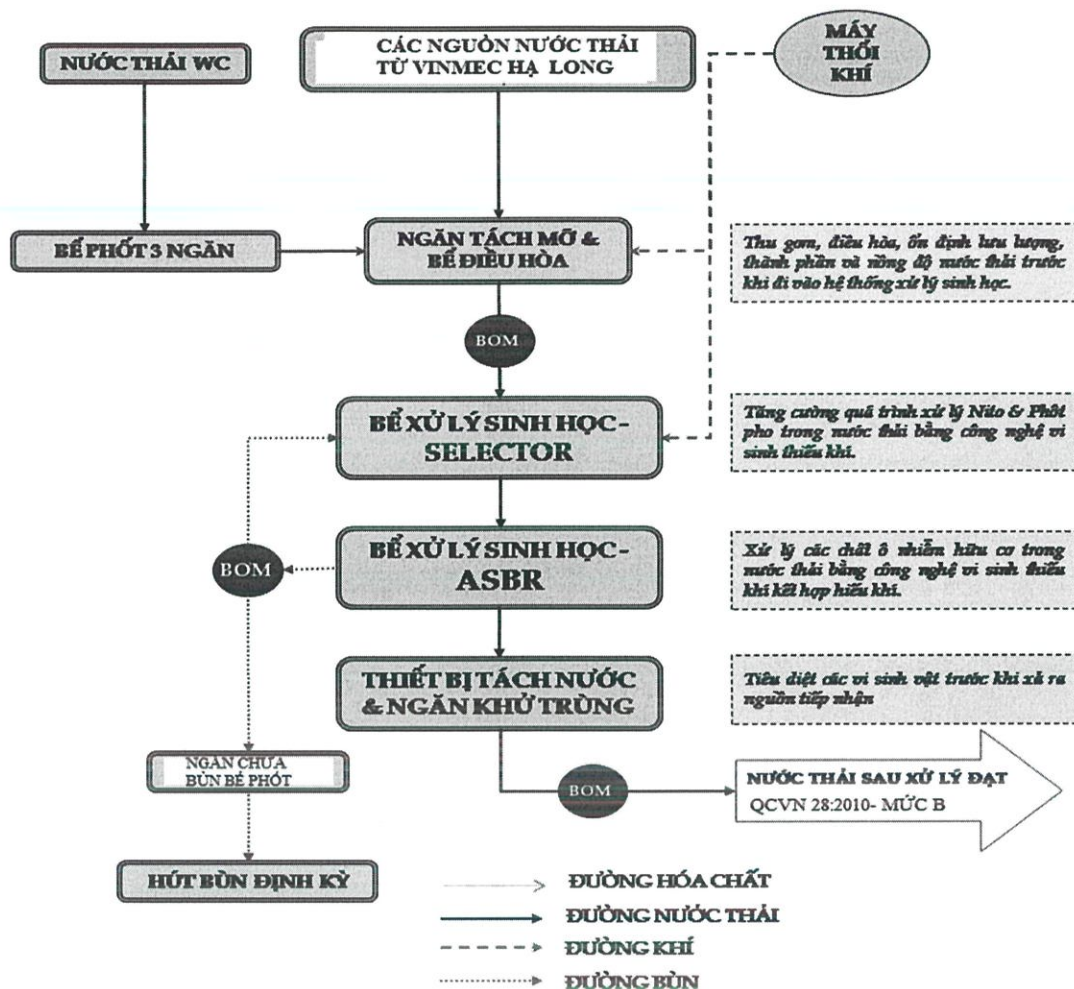
Hình 4. Sơ đồ dây chuyền quy trình công nghệ hệ thống xử lý nước thải Bệnh viện ĐKQT Vinmec Hạ Long
