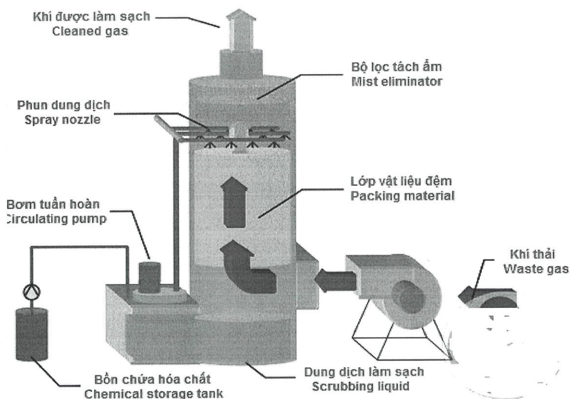
Hình 5. Nguyên lý tháp xử lý khí thải bệnh viện ĐKQT Vinmec Hạ Long
